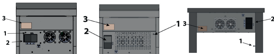
Obrázok 5. Pohľad na zadnú časť zariadenia
