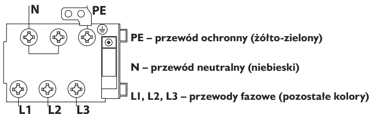
Rysunek 6. Podłączenie urządzenia do instalacji elektrycznej
