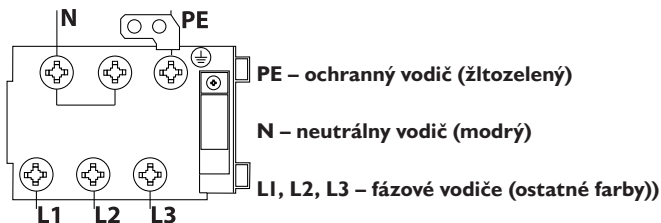
Obrázok 6. Pripojenie zariadenia k elektrickej inštalácii
