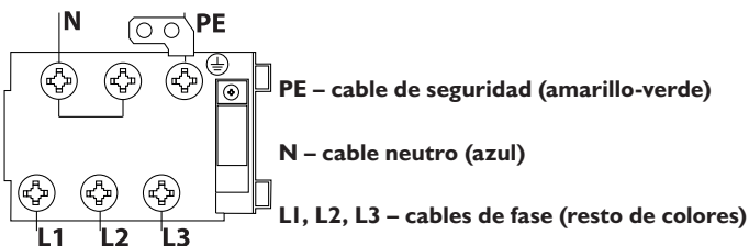
Figura 6. Conexión del equipo a la instalación eléctrica
