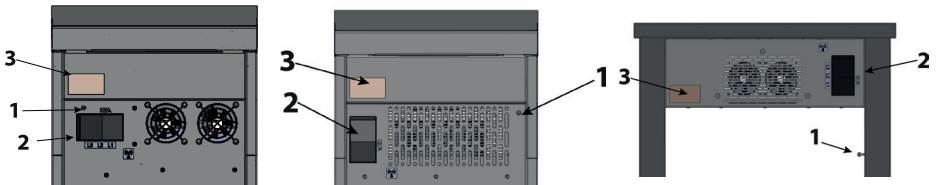
Figura 5. Vista trasera del dispositivo
