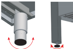
Rysunek 4. Poziomowanie urządzenia
