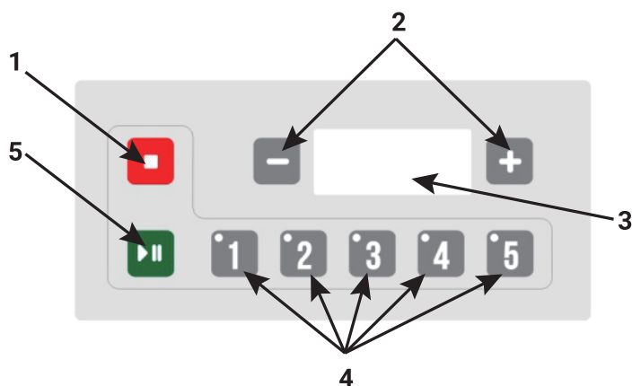
Abbildung 2 Bedienfeld
