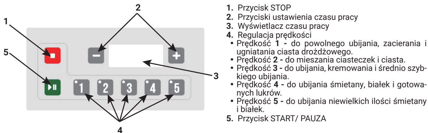
Rysunek 2. Panel sterowania
